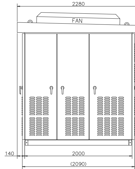
右側面図
