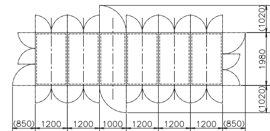
扉開閉図(尺度 1/100)
