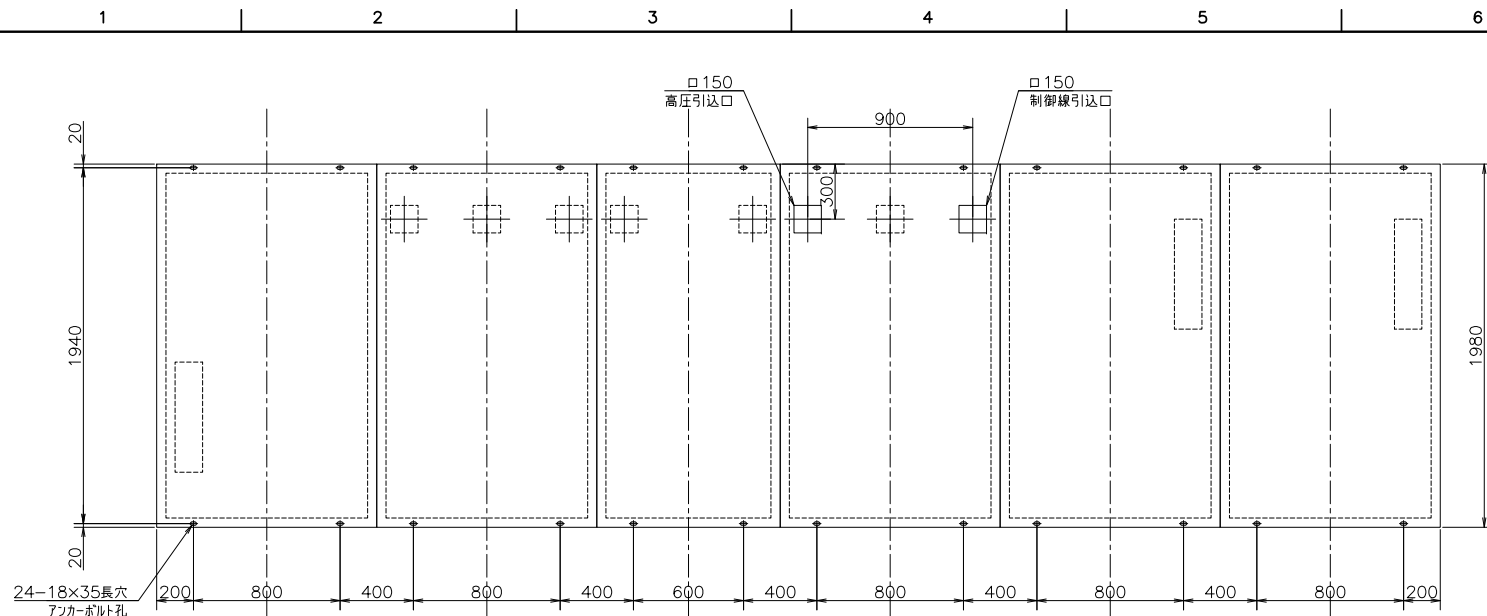
基礎図
