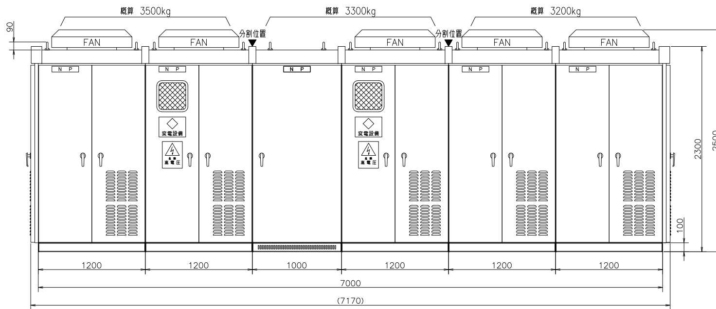
正面図
