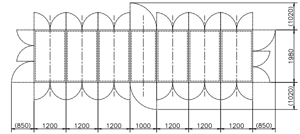
扉開閉図 (尺度 1/100)
